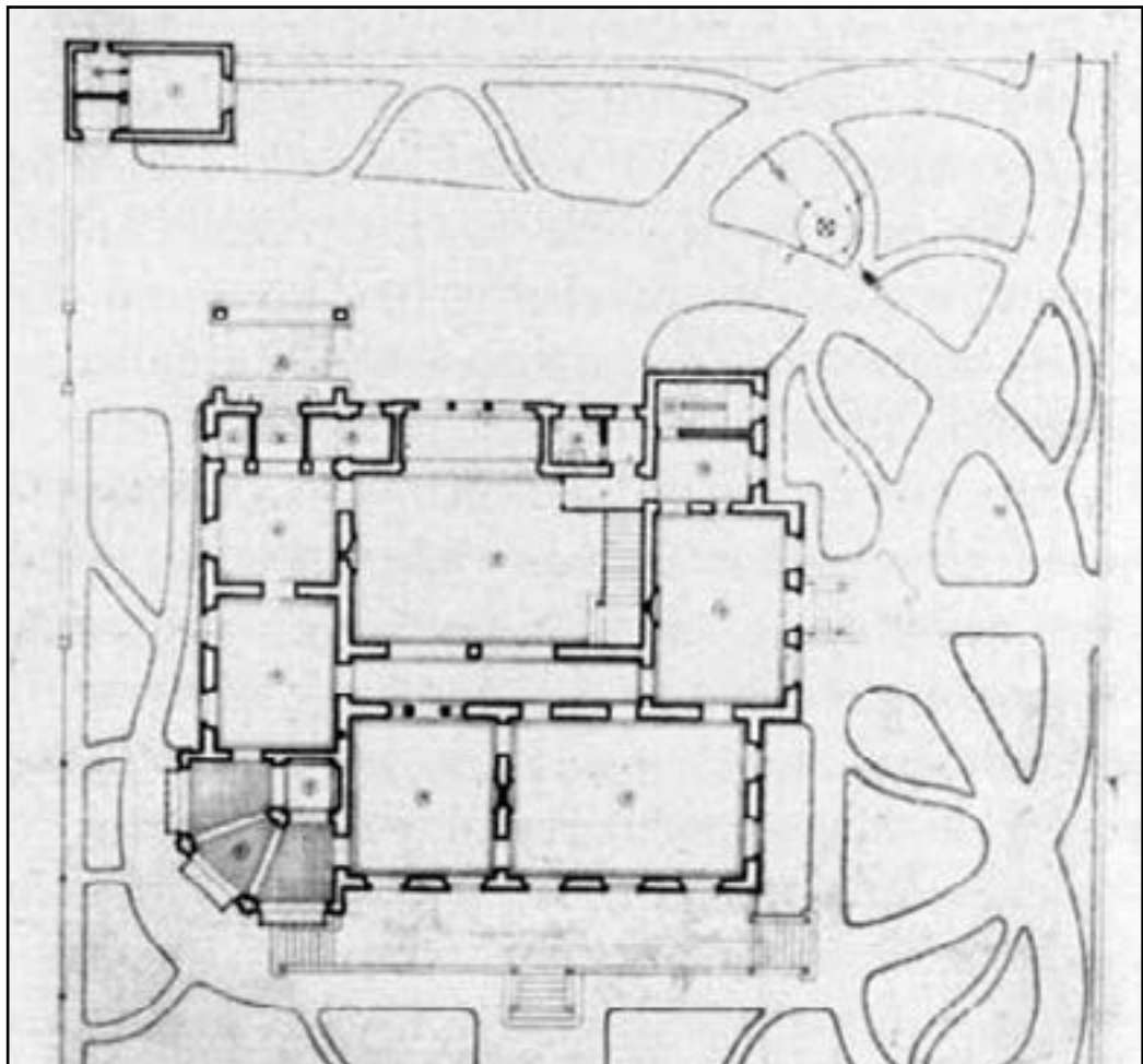
VILLA DELIELLA - PROSPETTO E PLANIMETRIA PIANO TERRA
